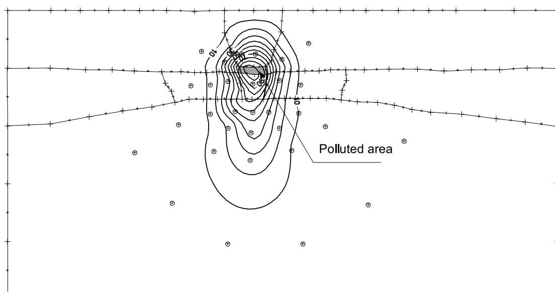
Obr. 6 Izolínie pomernej koncentrácie po 10 rokoch
