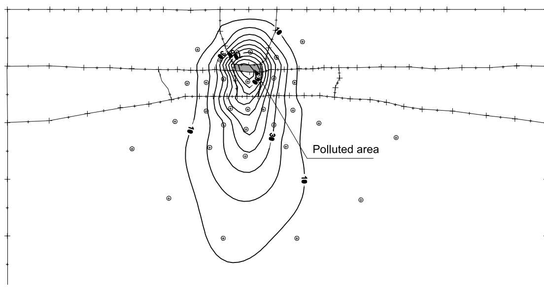
Obr. 7 Izolínie pomernej koncentrácie po 20 rokoch
