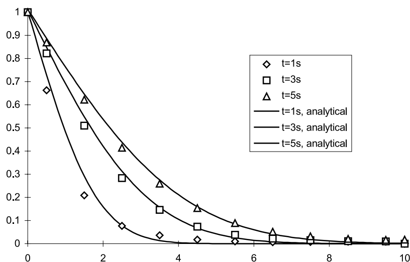
Obr. 4 Priebeh koncentrácie v jednorozmernom modeli
