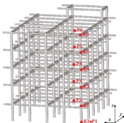
Fig. 9 FEM model render
