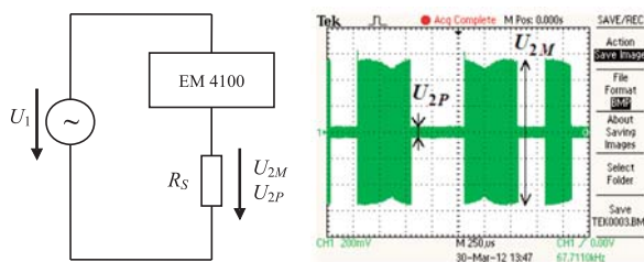
Fig. 3 Measurement of EM 4100 parameters
